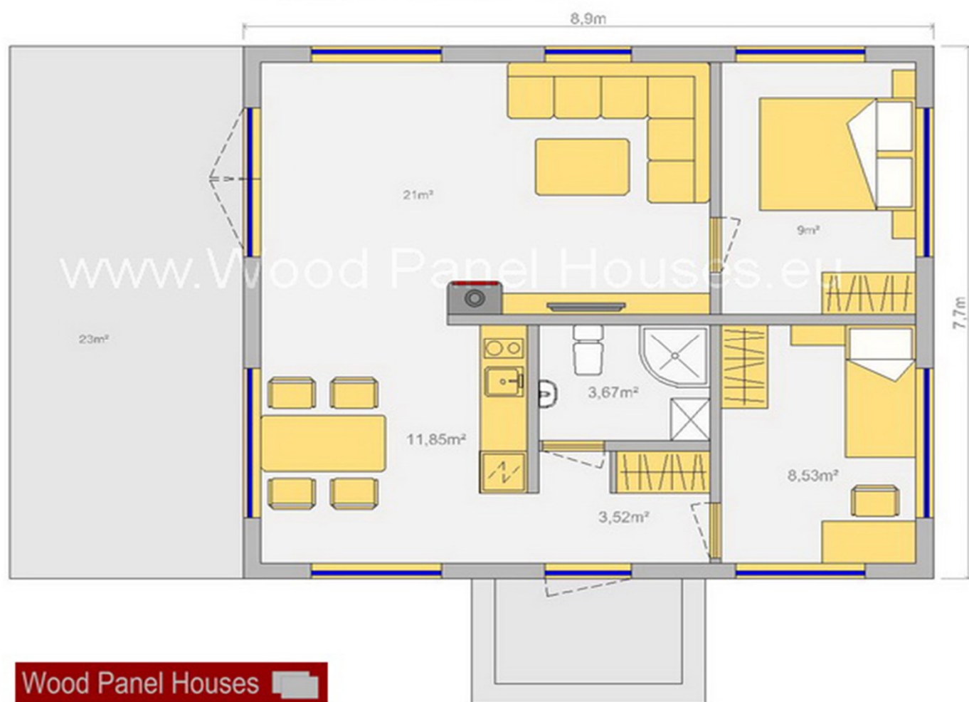
MOD_1_60_divu moduļu dzīvojamā māja_60m 2
